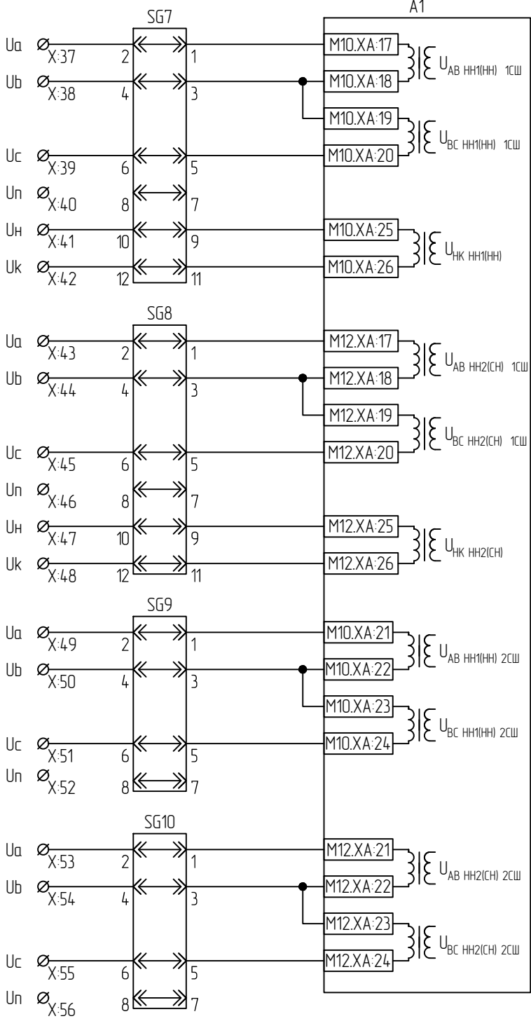
Цепи переменного и напряжения А1
